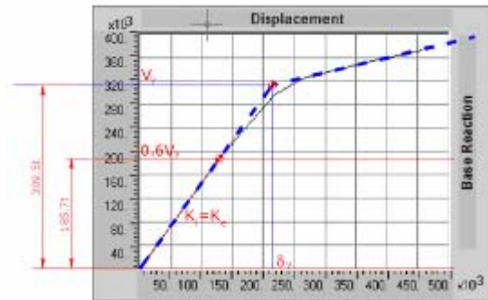
Gambar 17. Kurva Bi-linier Pushover arah X
