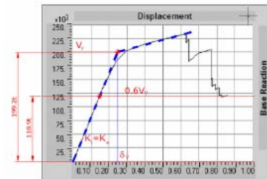
Gambar 18. Kurva Bi-linier Pushover Arah-Y
