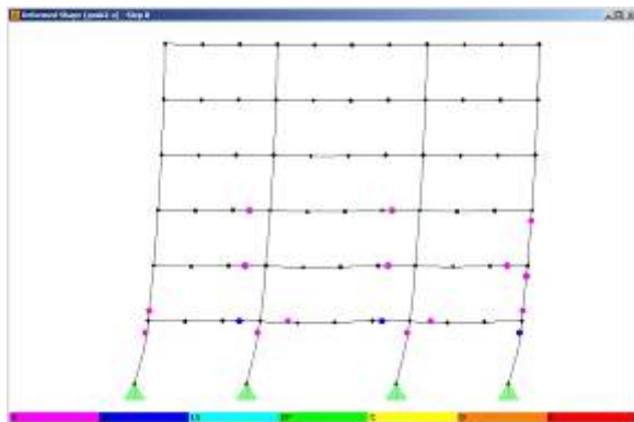
Gambar 21. Kinerja Struktur Arah X pada Step - 7
