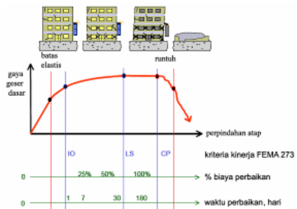
Gambar 1. Ilustrasi Rekayasa Gempa Berbasis Kinerja (ATC58)
