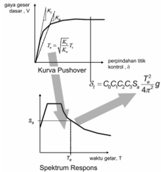
Gambar 4. Skematik Prosedur Metode Koefisien Perpindahan (FEMA 440)
