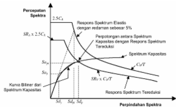
Gambar 5. Penentuan Titik Kinerja menurut Metode Spektrum Kapasitas
