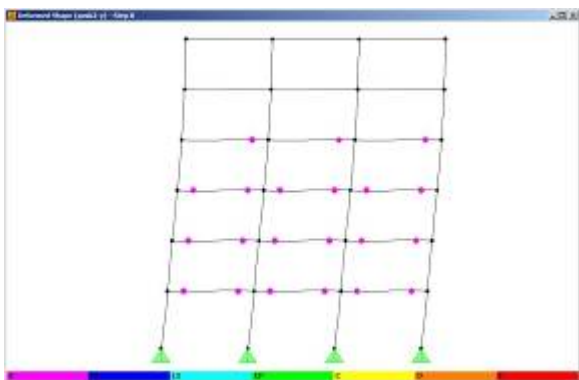
Gambar 22. Kinerja Struktur Arah Y pada Step - 5
