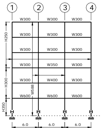
Portal A dan D
