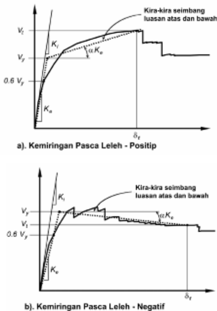
Gambar 3. Perilaku Pasca Leleh Sistem Struktur (FEMA 356)
