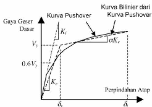
Gambar 2. Parameter Waktu Getar Fundamental Efektif dari Kurva Pushover
