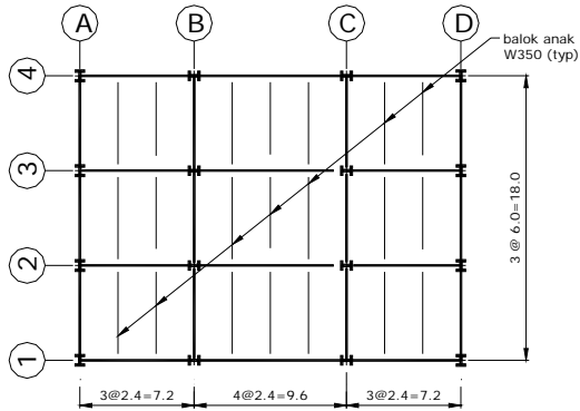
Gambar 8. Denah Bangunan Tipikal (m)
