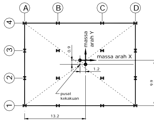
Gambar 11. Penempatan Massa dengan Eksentrisitas Rencana
