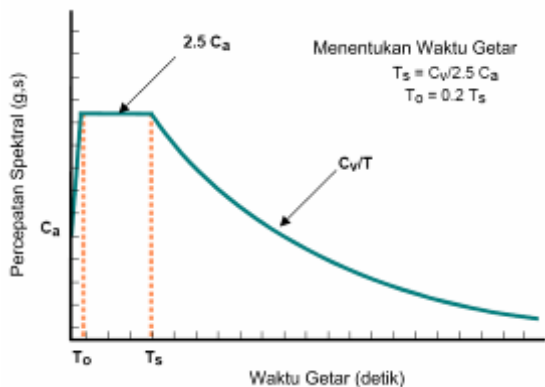
Gambar 6. Parameter data Respons Spektrum Rencana
