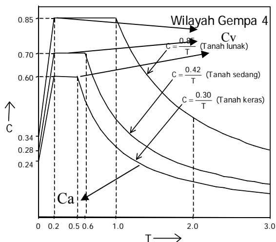
Gambar 12. Kurva Spektrum Respons Rencana (dari SNI - 1726 - 2002)
